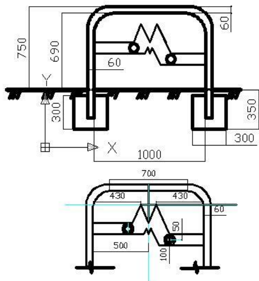
Схема модуля велостоянки
